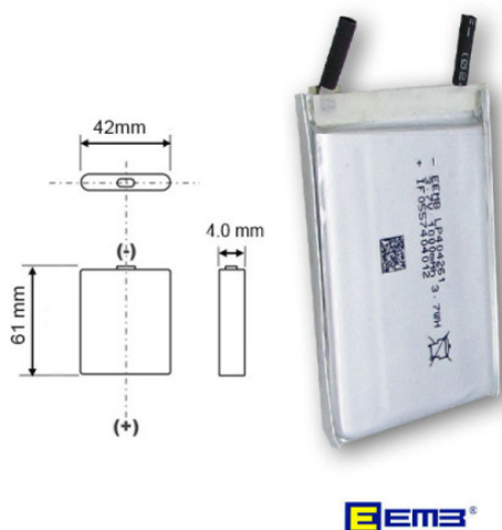
Li-Po LP404261 3.7V 1000mAh
